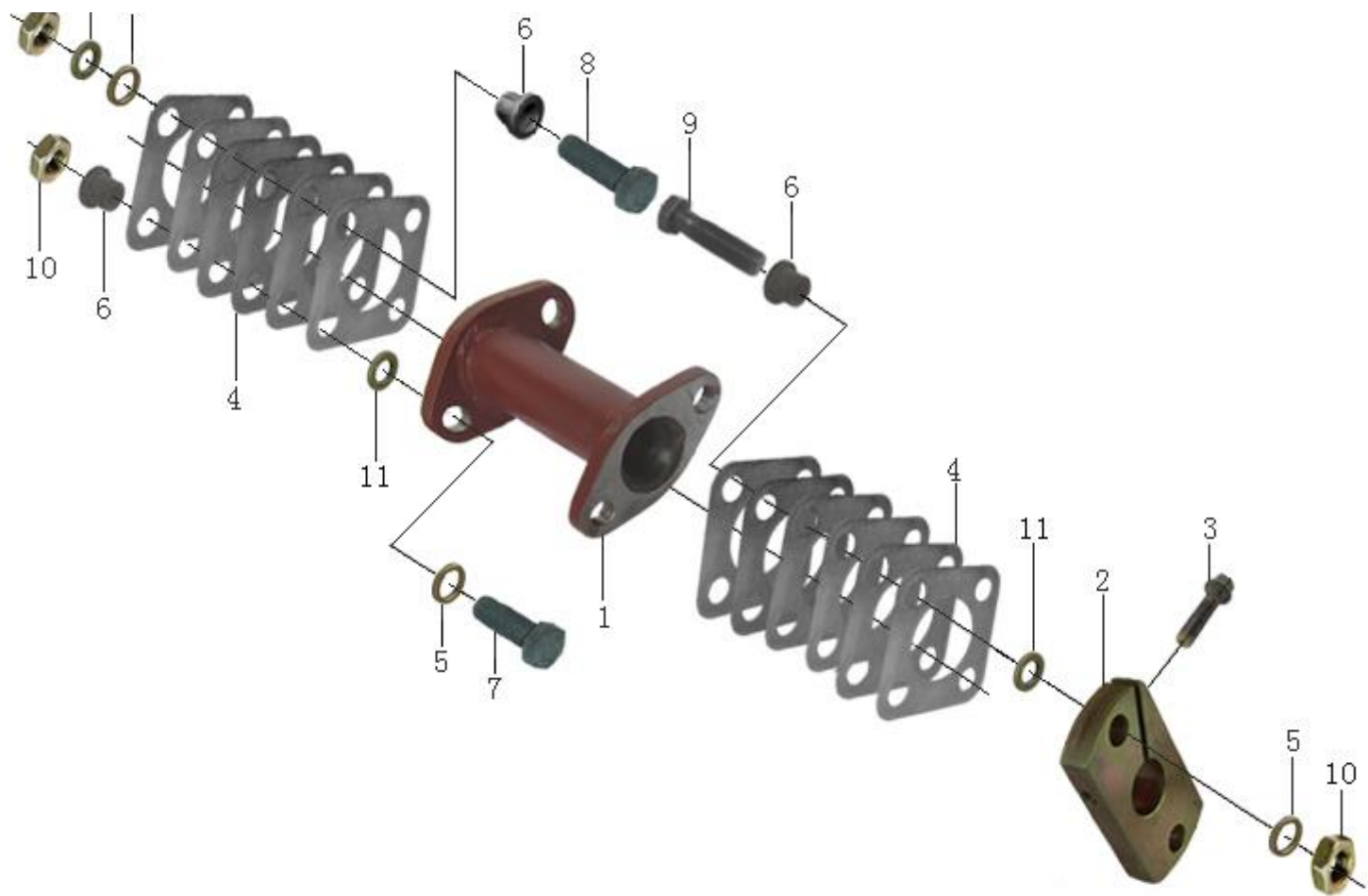
HW 发动机 FDJ15 联轴器
