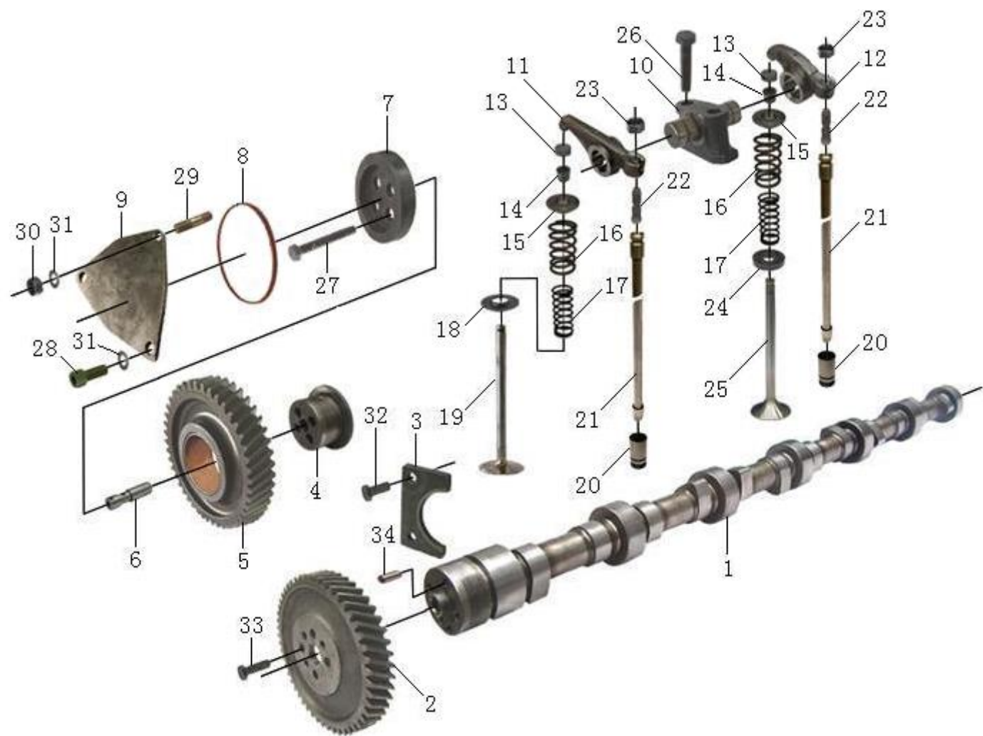
HW 发动机 FDJ07 配气机构
