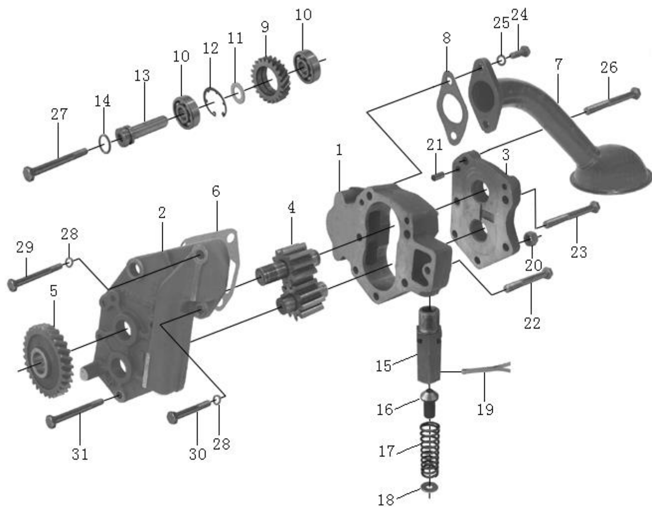
HW 发动机 FDJ11 机油泵
