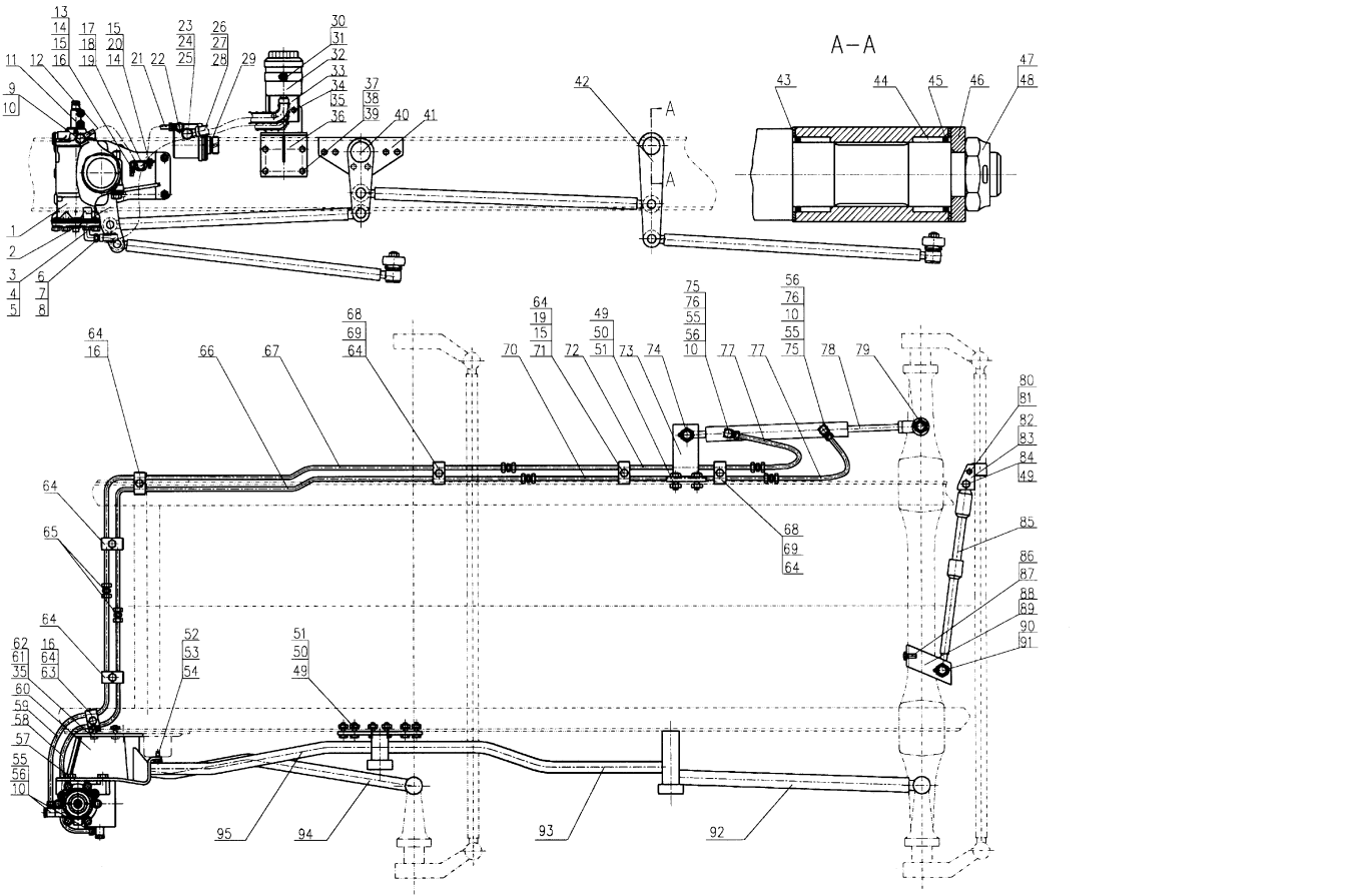
微压动力转向系统 (8×4)
