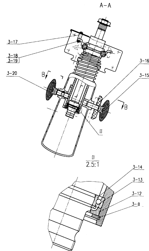
转向轴带管柱总成
