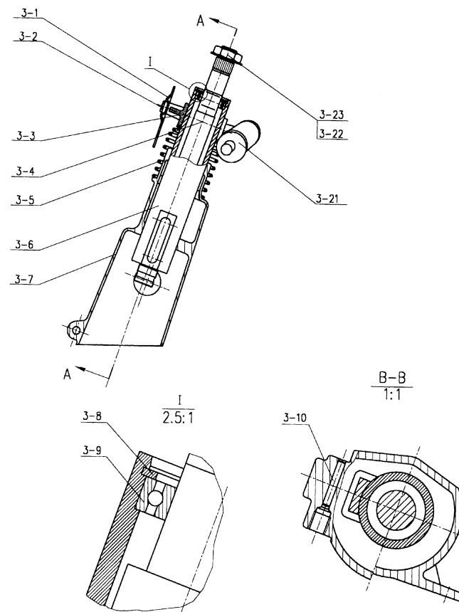
转向轴带管柱总成
